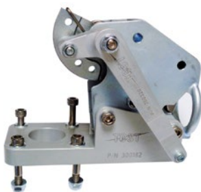
Adapterbeschlag KT 12
