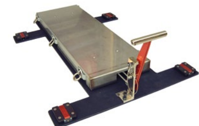
6-Mann-Abseilsicherung
