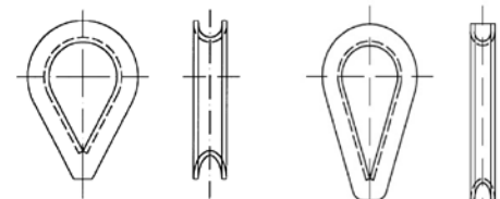
Herzkausche
