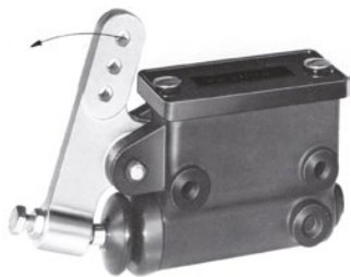
Universal-Hauptbremszylinder Form 4
