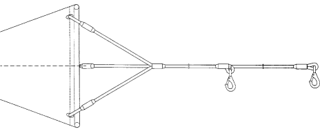
Treibanker
