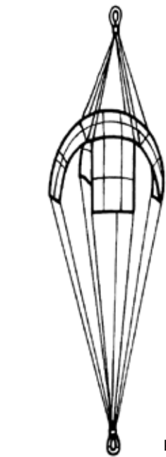
Kreuzbahnschirm Kuwi für Kunststoffseile
