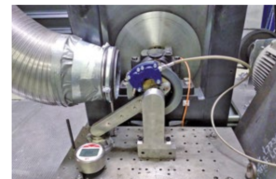
Bremstest mit Massenschwungrad zur Ermittlung der Bremsleistung
