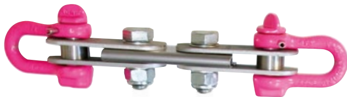
Vierteiliges Lastsollbruchelement in Einzelschaltung
